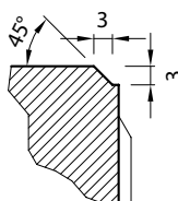
Řez hranou
