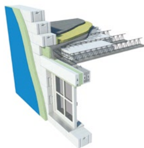
Vizualizace skladby nosných a nenosných překladů při tloušťce stěny 375 mm.
