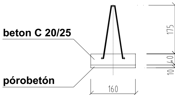
Stropní nosník PORFIX – řez
