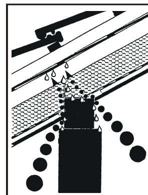
13 b/ Detail v oblasti uložení krokvi na vaznici nebo mezistěny v konstrukci větrané střechy: parotěsné a vzduchotěsné vrstvy nejsou funkčně napojeny
