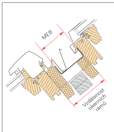
Řez okny R4/R7
