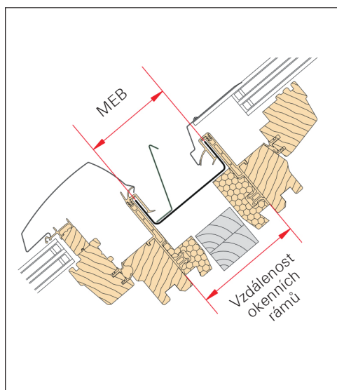
Řez okny R6/R8
