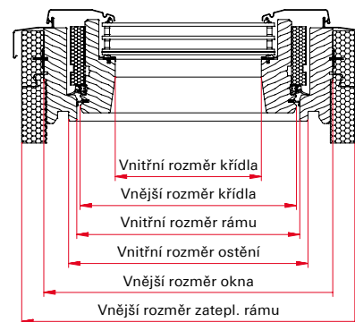
řez B-B
